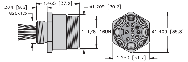
"C" P-RSF .. M20
