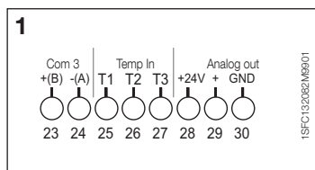
Figura 1: Conexión de terminales
