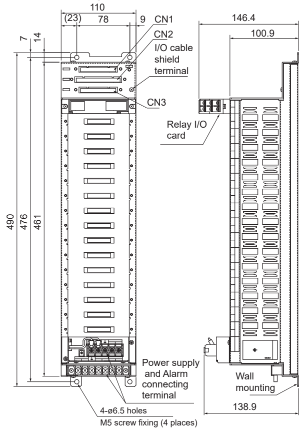
AC Power Supply (RVV-11, RVV-21)
